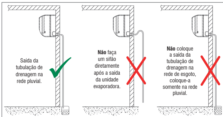
FIG. 8 - EXEMPLOS DE SITUAÇÕES DE DRENAGEM
