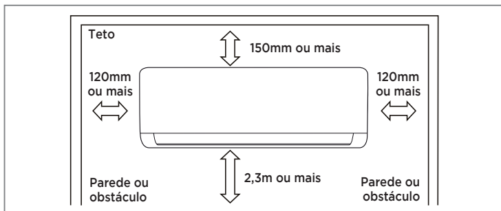
FIG. 7 - ESPAÇAMENTOS MÍNIMOS RECOMENDADOS
