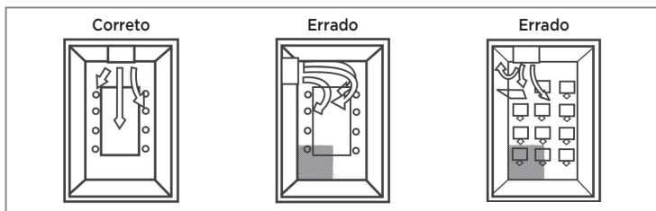
FIG. 6 - POSICIONAMENTO DA UNIDADE EVAPORADORA NO AMBIENTE
