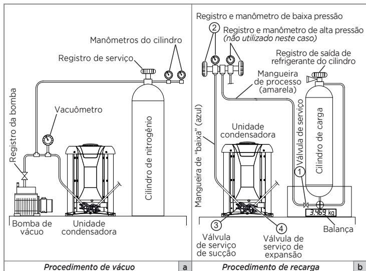
FIG. 16 - PROCEDIMENTOS DE VÁCUO E RECARGA
