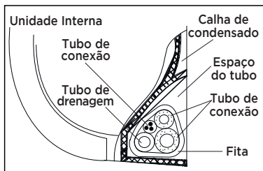
FIG. 9 - TUBO DE CONEXÕES
