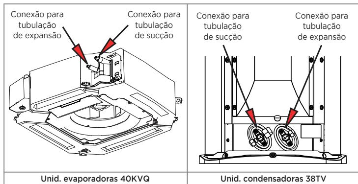
FIG. 31 - CONEXÕES DE INTERLIGAÇÃO
