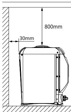
FIG. 2 - UNIDADE CONDENSADORA 38TV
