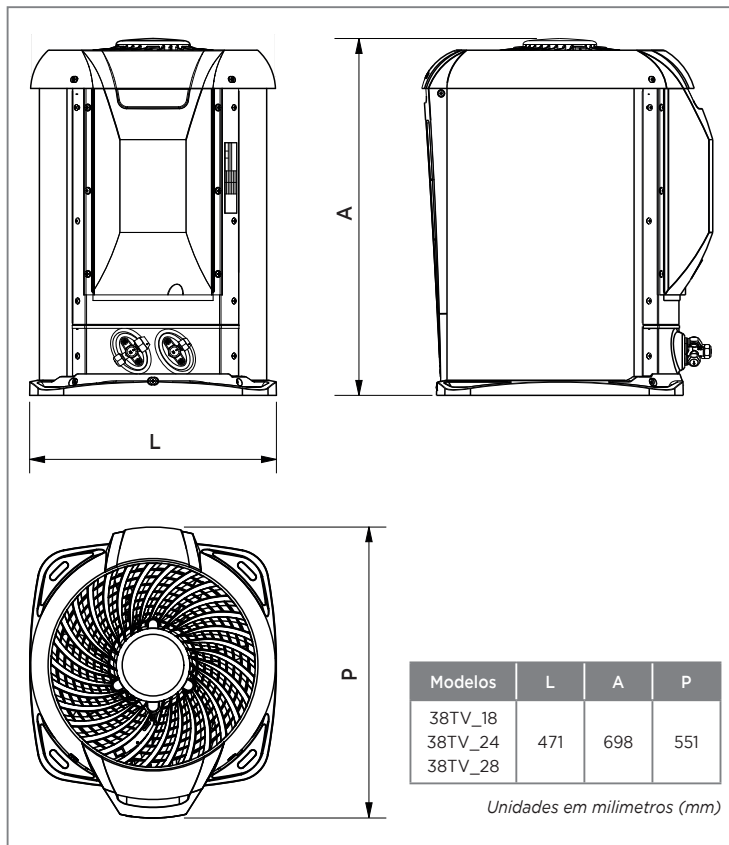
FIG. 9 - DIMENSIONAIS
