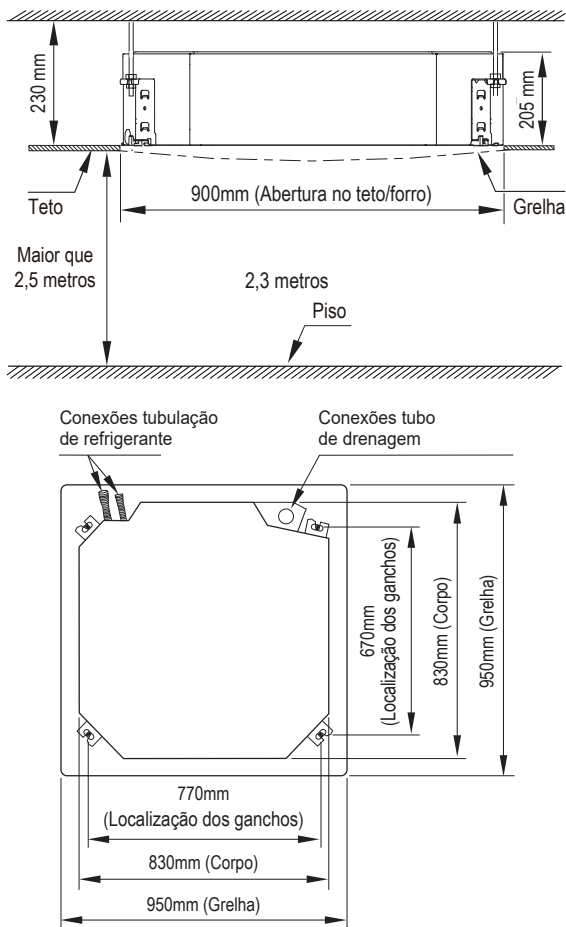
FIG. 12 - DIMENSIONAL E ESPAÇAMENTOS MÍNIMOS
