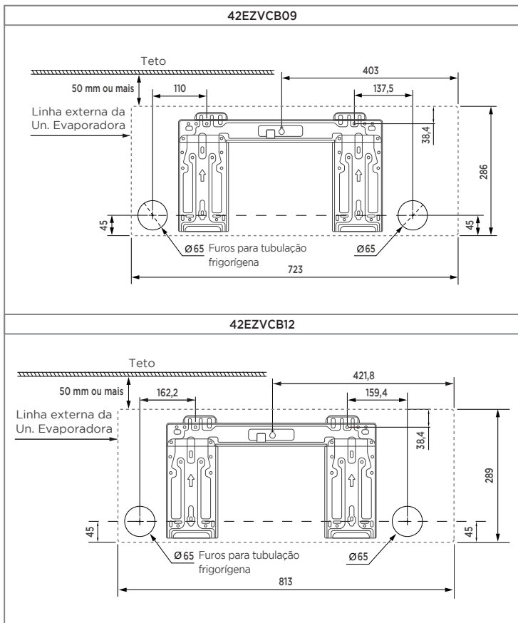
FIG. 11 - SUPORTES DE MONTAGEM
