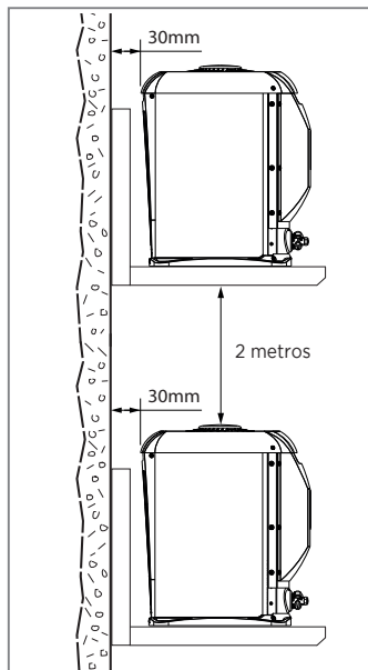
FIG. 6 - INSTALAÇÃO COM MÃO-FRANCESA
