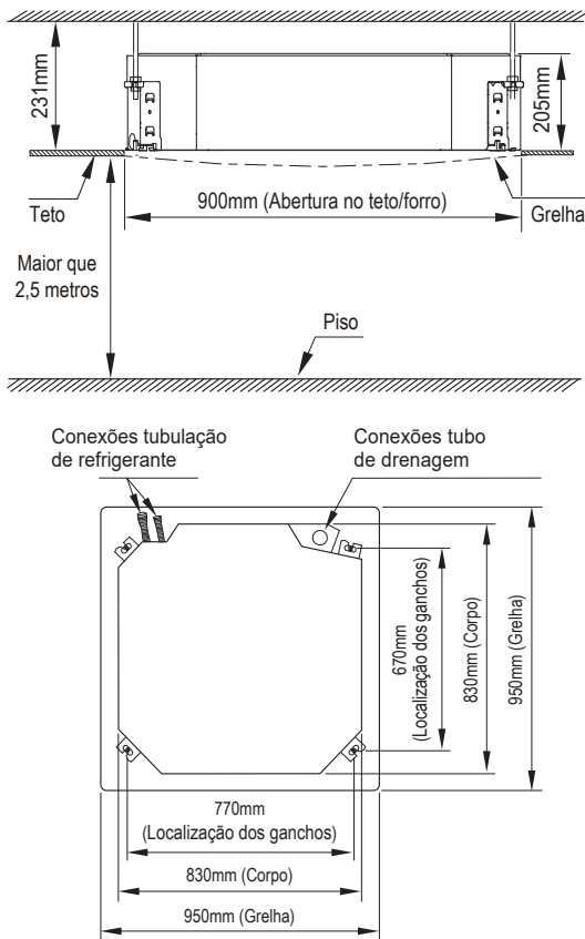
FIG. 12 - DIMENSIONAL E ESPAÇAMENTOS MÍNIMOS
