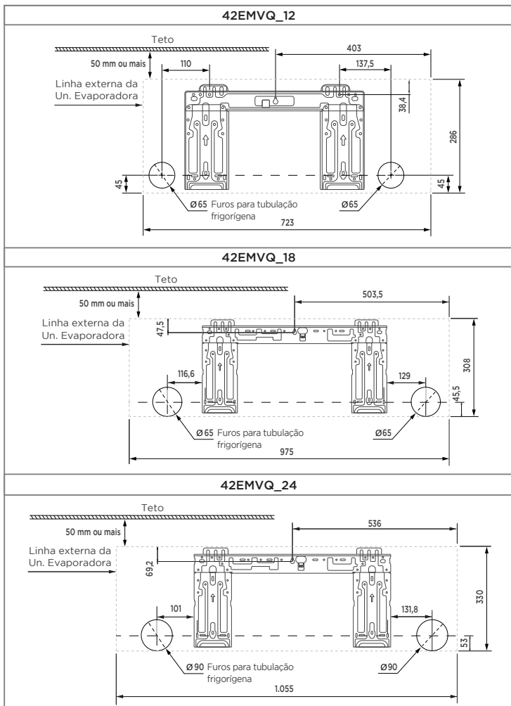
FIG. 11 - SUPORTES DE MONTAGEM
