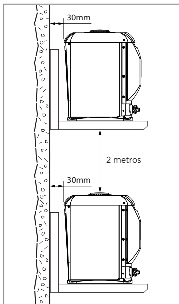
FIG. 5 - INSTALAÇÃO COM MÃO-FRANCESA
