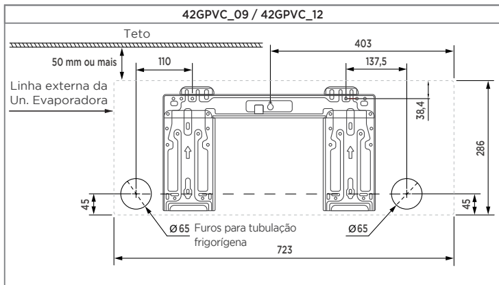
FIG. 18 - SUPORTES DE MONTAGEM
