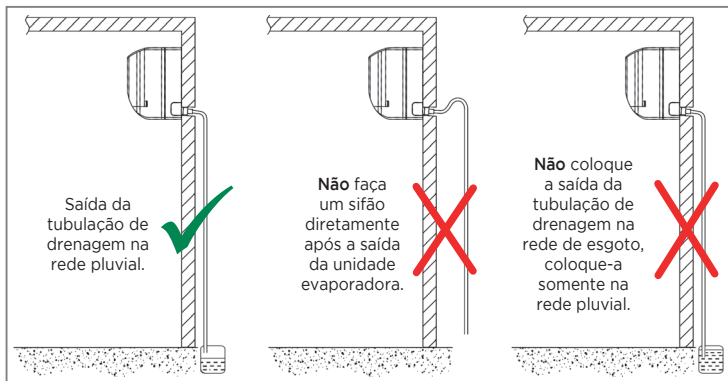
FIG. 14 - EXEMPLOS DE SITUAÇÕES DE DRENAGEM
