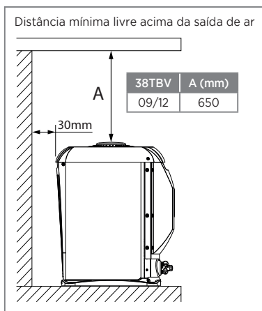
FIG. 1 - UNIDADE CONDENSADORA 38T
