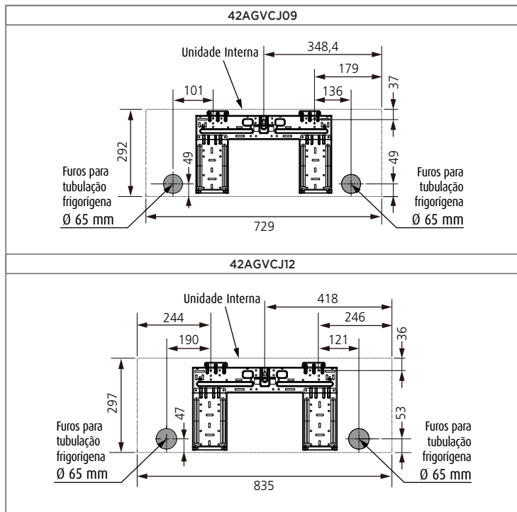
FIG. 11 - PLACAS DE MONTAGEM
